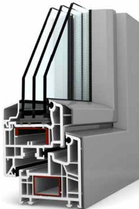
SOFTLINE70 ALU SCHALE mit 3-fach-Verglasung
